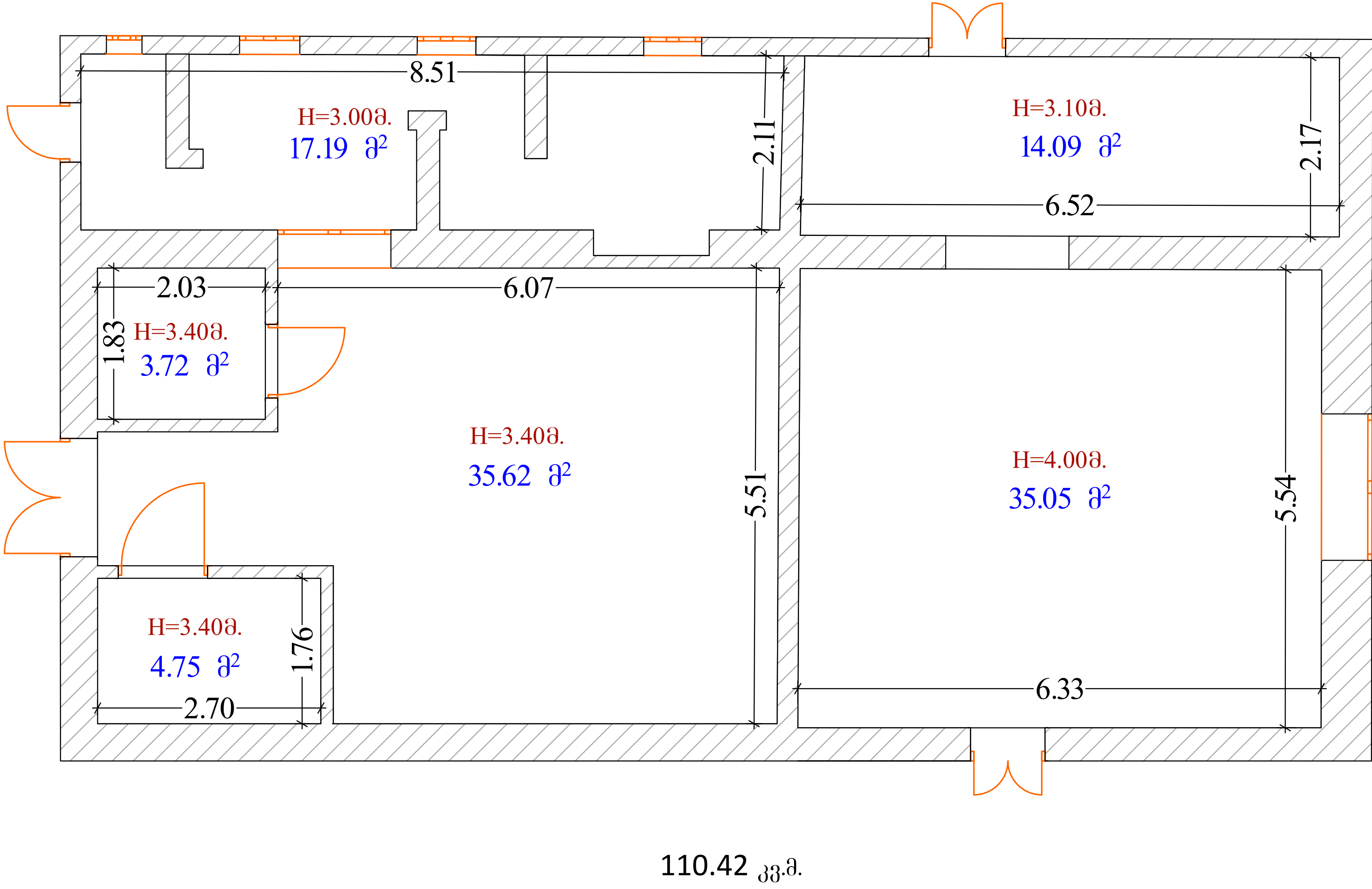
№8 პრტ სართულიანი შენობა-ნაგებობის გეგმა
