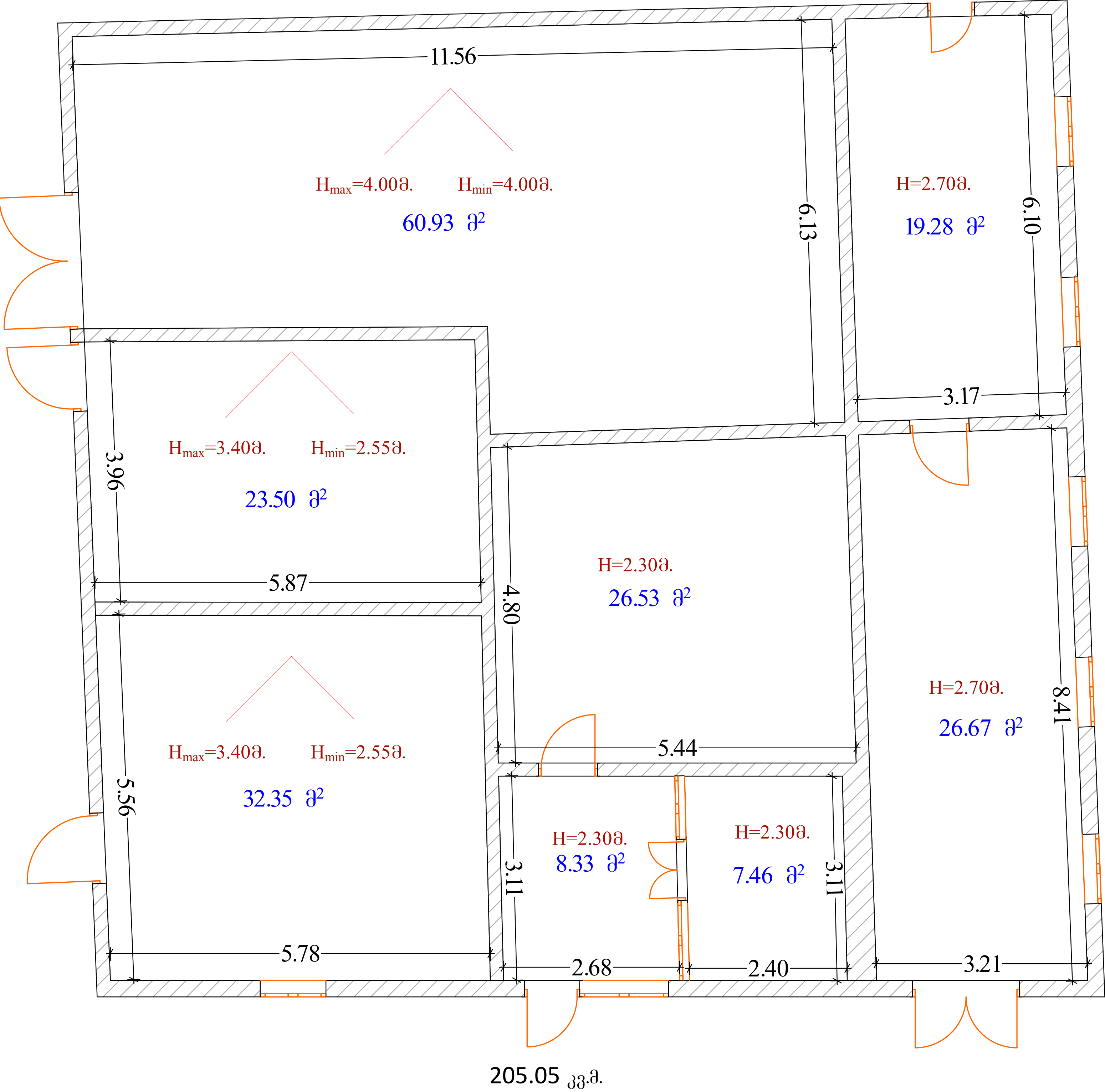
№9 პრტ სართულიანი შენობა-ნაგებობის გეგმა
